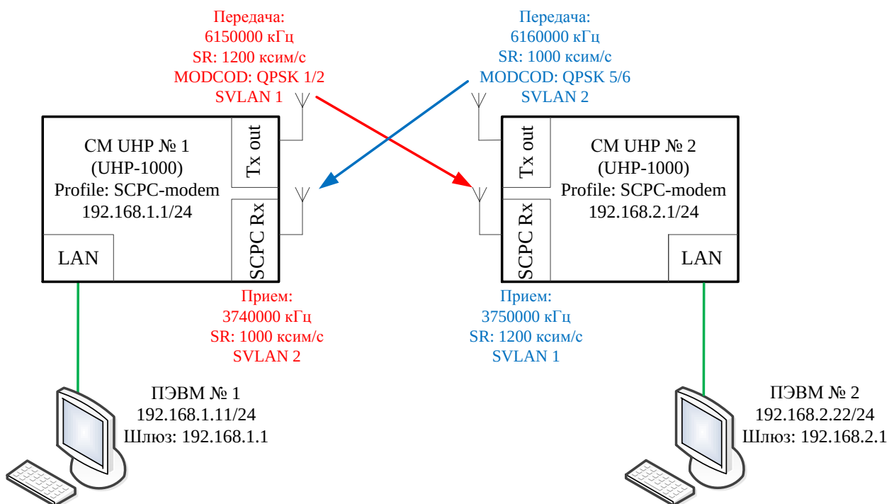
Рисунок 1. Сеть топологии «точка-точка», построенная на СМ UHP-1000 в составе ЗССС С-диапазона
